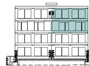
Façade est
